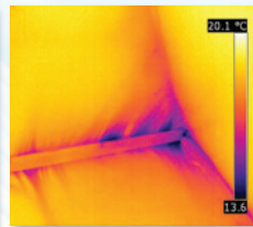
Exakte Thermografie einer Luftleckage während des BlowerDoor Tests
