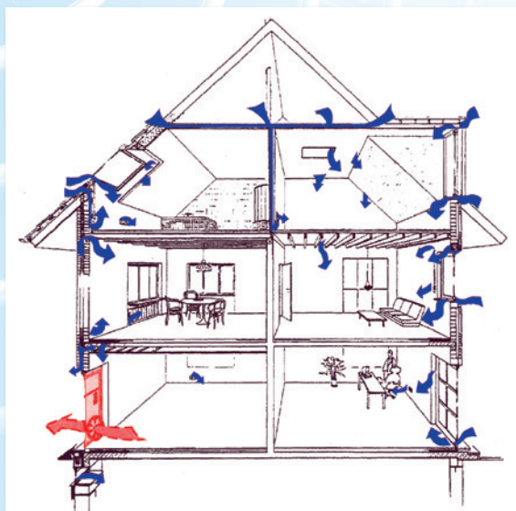
Das Prinzip der BlowerDoor Messung: Ein Ventilator saugt Luft aus dem Gebäude. Außenluft strömt durch undichte Stellen ins Gebäudeinnere.
