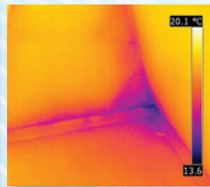
Thermogramm einer Luftleckage
